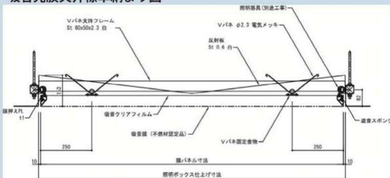
吸音光膜天井標準納まり図
