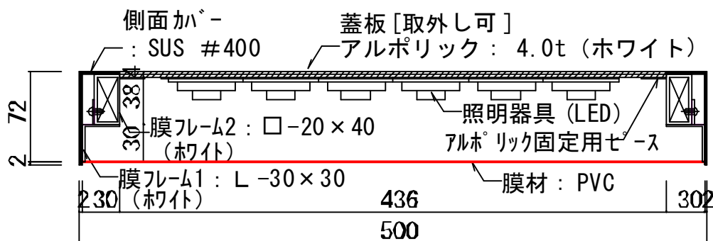
断面詳細図
