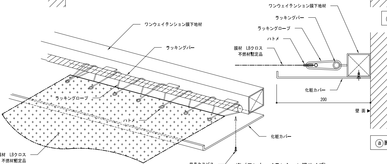
(a) 断面図
